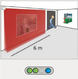
Por el día, solo el campo 1 está activado y acciona el relé 1.
