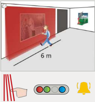
Campo 1 (4 cortinas activadas) acciona el relé 1: Advertencia.
